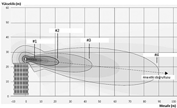
20 metre civarında yüksekliğe sahip bir binaya yerleştirilmiş baz istasyonu anteninin yönlü yaptığı ana ışıma lobu
